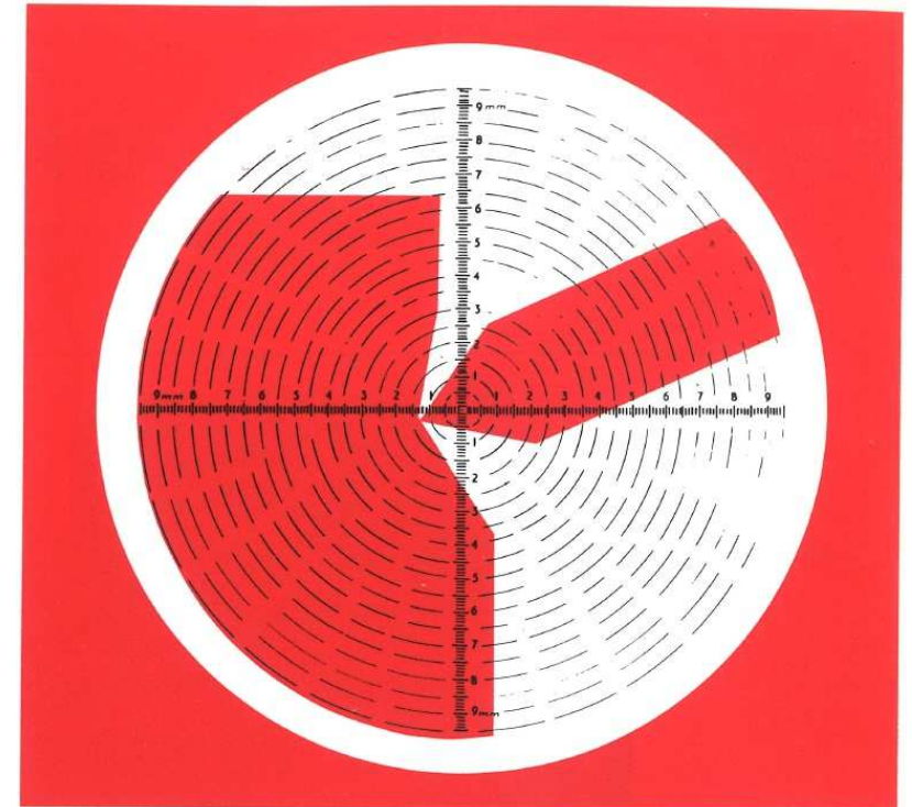
マイクروسコープの目盛板上に投影された砥石とダイヤモンドツール
